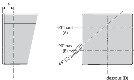
Sorties manivelle
