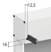
Sortie sur face avant
