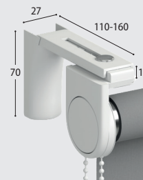
P4 Équerre de déport A Déport de 57 à 107 mm. Guidage impossible.
